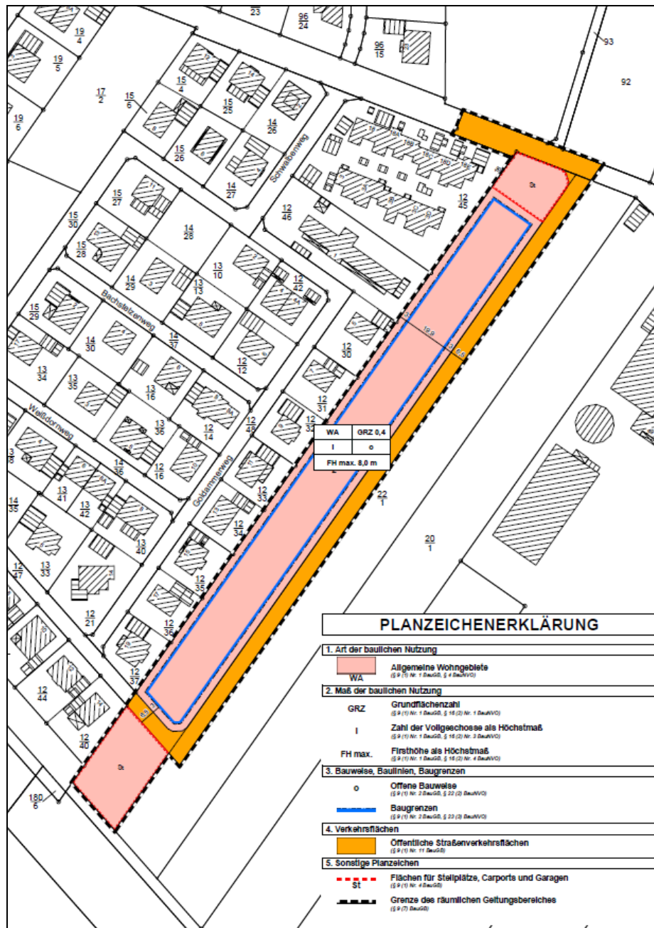
Abbildung 1 Vorentwurf des Bebauungsplanes, Stand 05.08.2025
