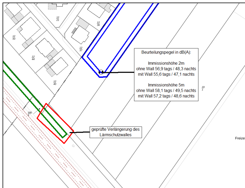
Abbildung 2 Prüfung Verlängerung Lärmschutzwall
